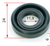
Código: 3710 Quant. 01 Retentor do alternador Bosch Spinter S10 / Ranger (com bomba de óleo).
