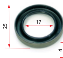
Código: 3714 Quant. 01 Retentor do alternador Bosch Wapsa ônibus MB 75 ampères (sem mola).
