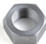
Código: 1647B Quant. 10 Porca do alternador Marea/Magneti Marelli. M17 rosca esquerda.
