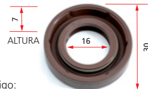
Código: 3758 Quant. 01 Retentor alternador L200 Kia com bomba vácuo 12v.
