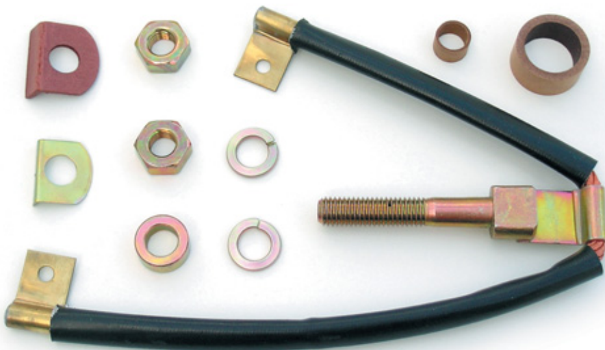
Código: 0386 Quant. 01 Conexão da partida KB / MWM / CUMMINS Bosch – marítimo.
