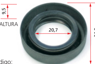
Código: 3724 Quant. 01 Retentor da partida Delco Remy 50MT caminhão VW / Ford.
