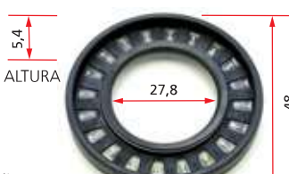
Código: 3727 Quant. 01 Retentor da partida Mitsubishi.
