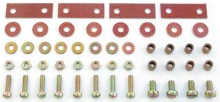
Código: 0346 Quant. 01. Rep. da part. portaescovas MB KB p/ 4-escovas positivas isolantes.
