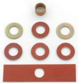
Código: 1856 Quant. 01. Reparo da partida MB JF (só isolantes).
