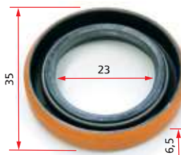
Código: 3716 Quant. 01 Retentor da partida Delco Remy 37MT CUMMINS VW / Ford (com mola).
