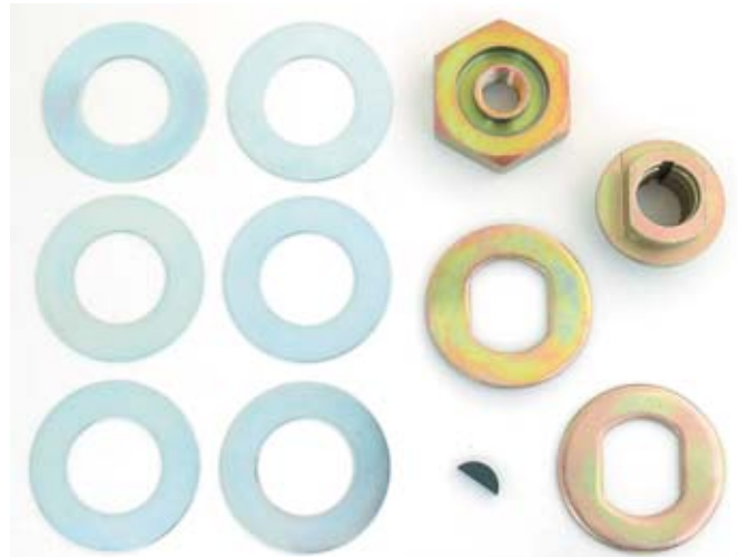
Código: 2005 Quant. 01. Reparo de fixação da ventoinha dínamo e alternador VW / Brasília / Kombi.
