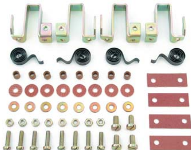
Código: 0349 Quant. 01. Reparo da partida portaescovas MB KB Bosch (4-escovas positivas).
