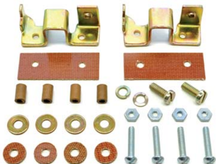
Código: 0351 Quant. 01 Reparo da partida portaescovas Valmet.
